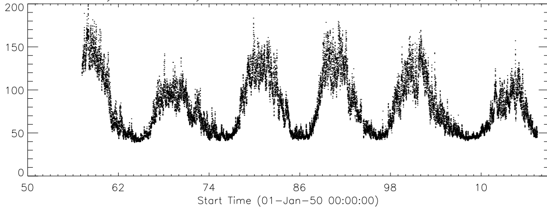
2GHz (sfu)
