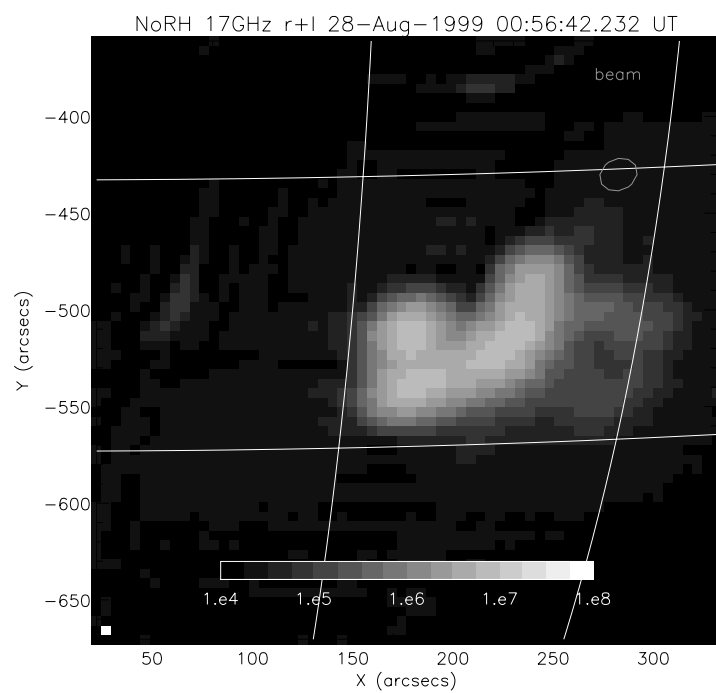
图 2: 17GHz (R+L) 画像
