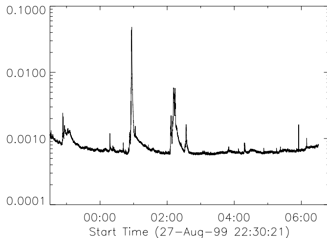
図 1: 光度曲線 ( 相関値プロット )
