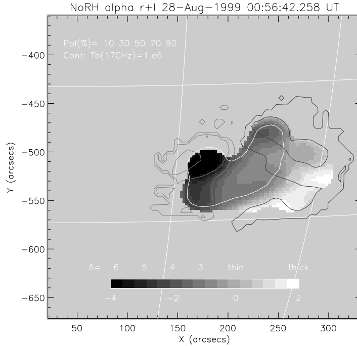
図 4: スペクトルグラム (グレースケール) T_b^{17\text{GHz}} = 1\text{MK} の等高線 (太線) 偏波率等高線 (細線)
