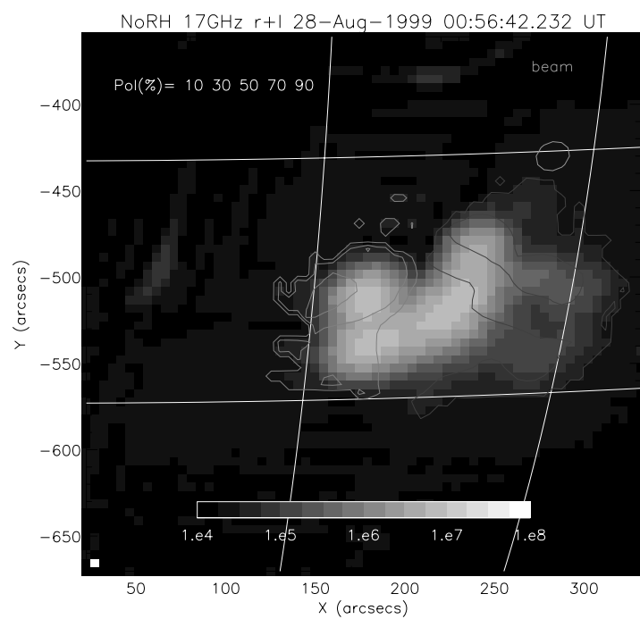
图 3: 17GHz 円偏波率画像
